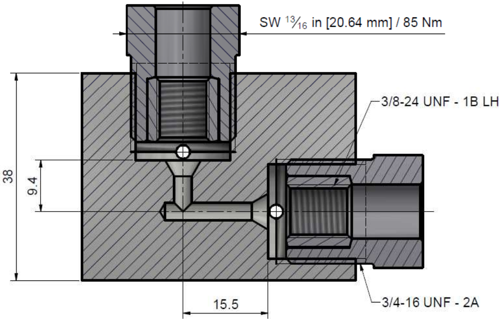
Schnitt A-A ( 2 : 1 )
