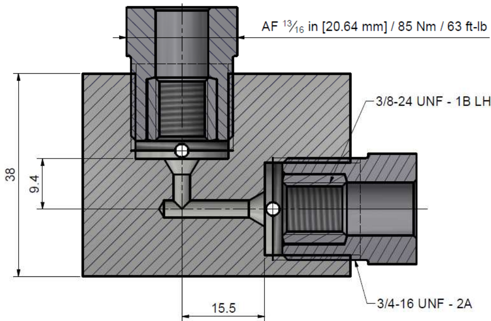
Schnitt A-A ( 2 : 1 )
